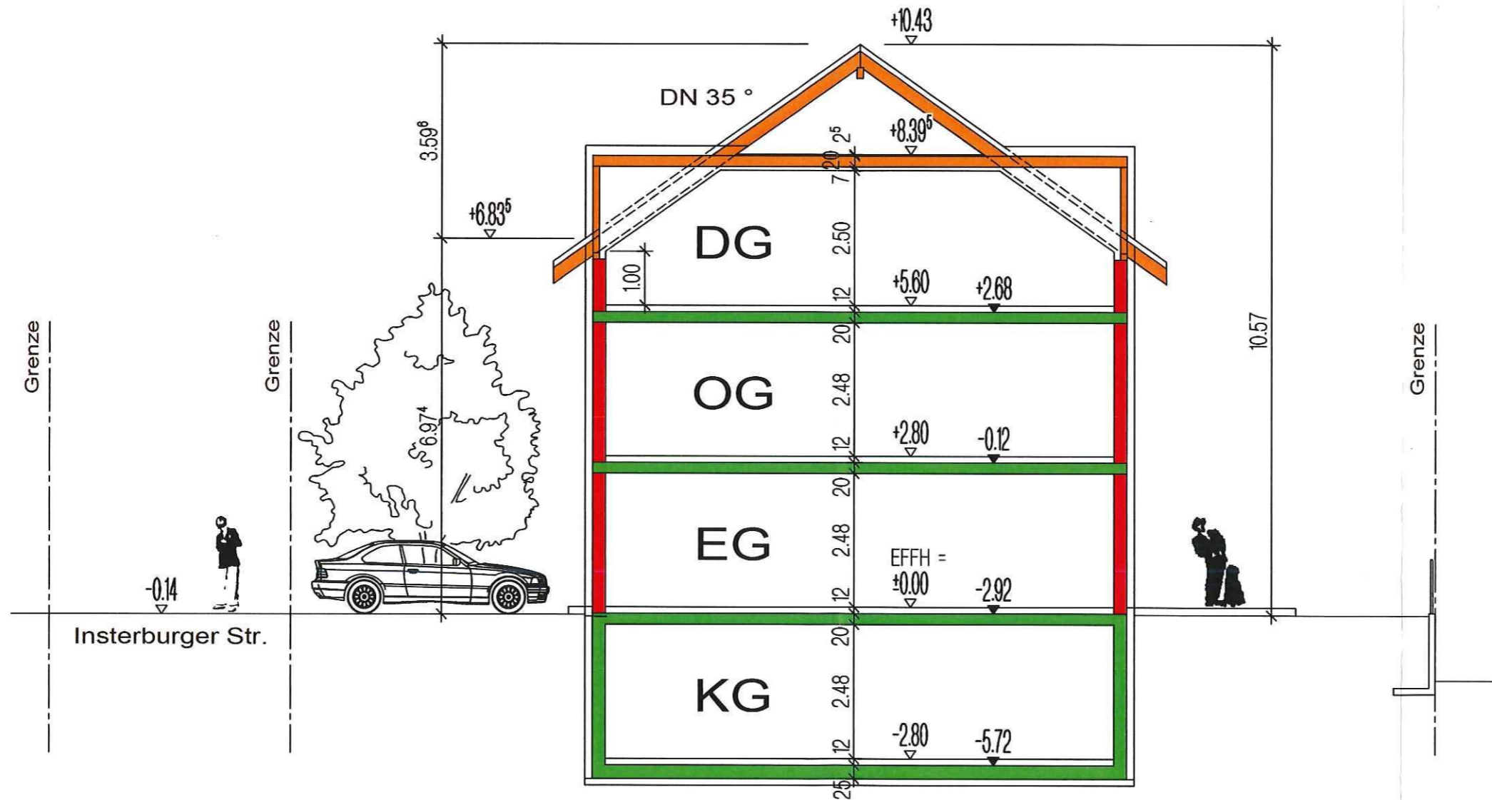
Systemschnitt Doppelhausbebauung
