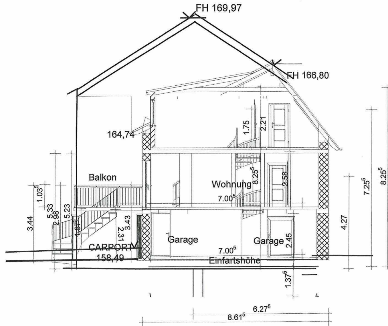
Schnitt C--C
