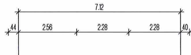
Ansicht Süd-Ost
