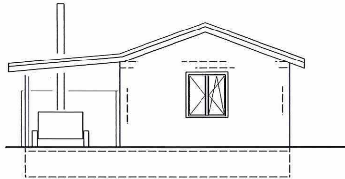
Ansicht Süd-Ost
