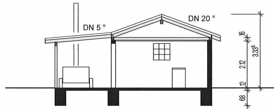
Schnitt A-A
